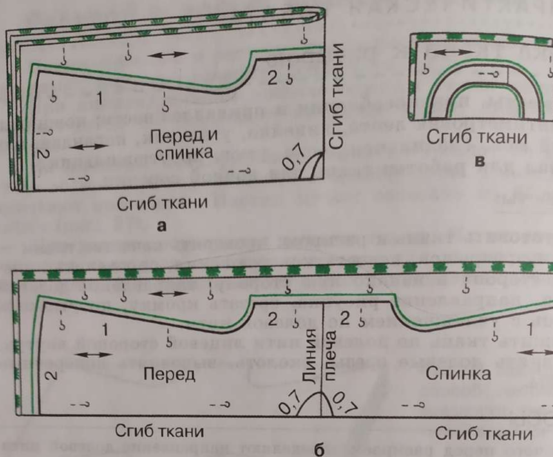
Рис. 29. Варианты раскладки на ткани: а, б — раскладка деталей выкройки сорочки; в — раскладка выкройки обтачки
